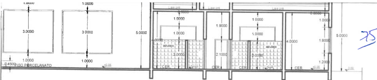
CORTE TRANSVERSAL esc. 1/100
